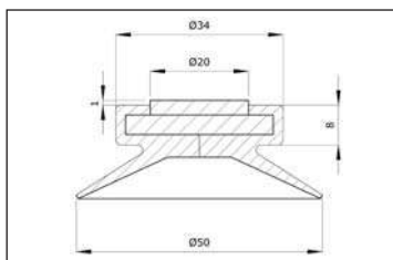
Maße nach DIN 16901
